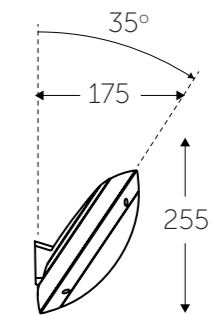
REMI LUCÍA 10 W CÓN MÓDULO E27 23 W MÁXIMO
