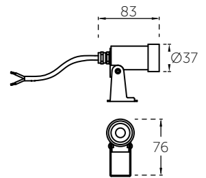
HOUSING PARA EMPOTRAR ACCESORIO REQUERIDO NO INCLUIDO
